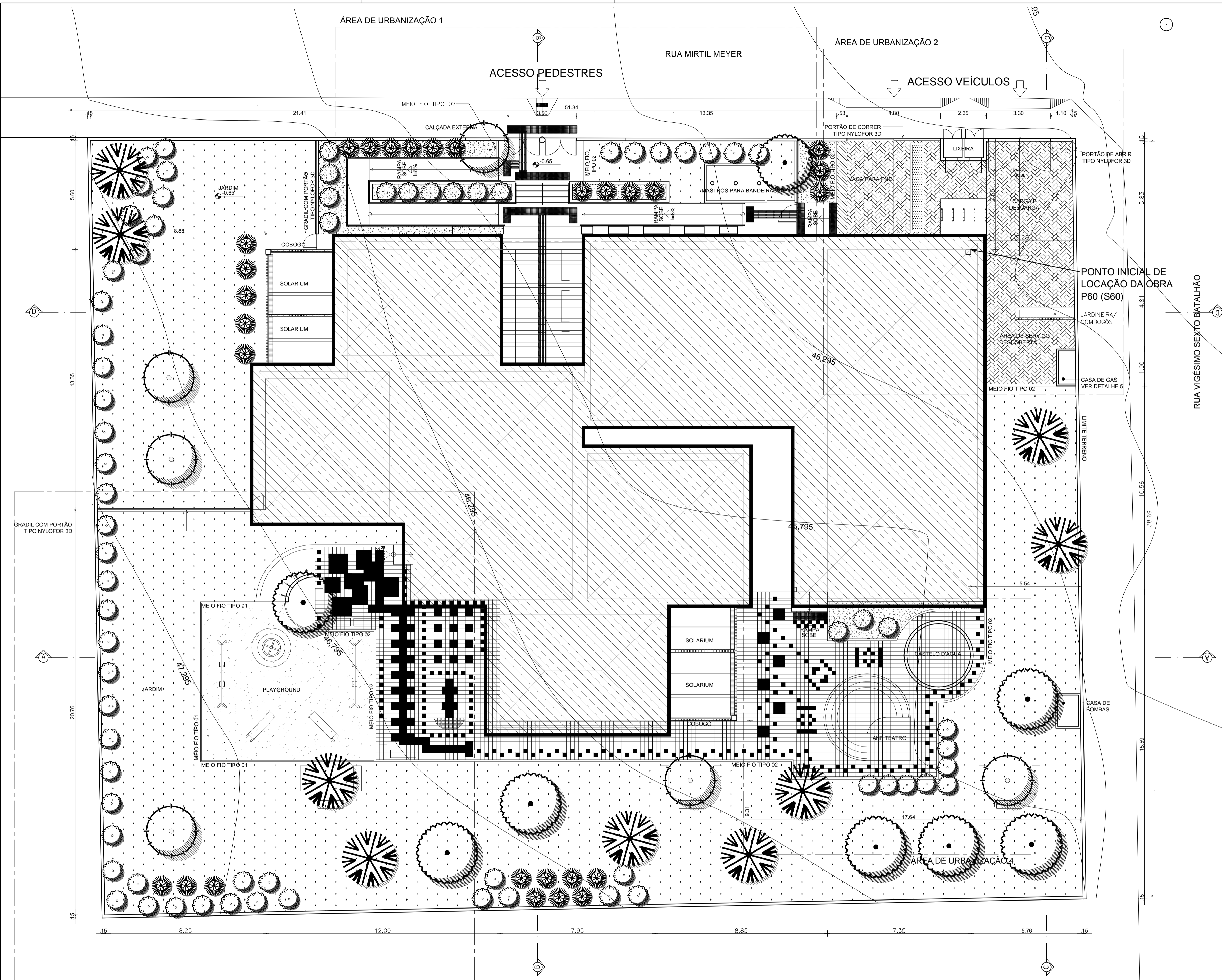
01 PLANTA DE PAISAGISMO ESCALA: 1:100
